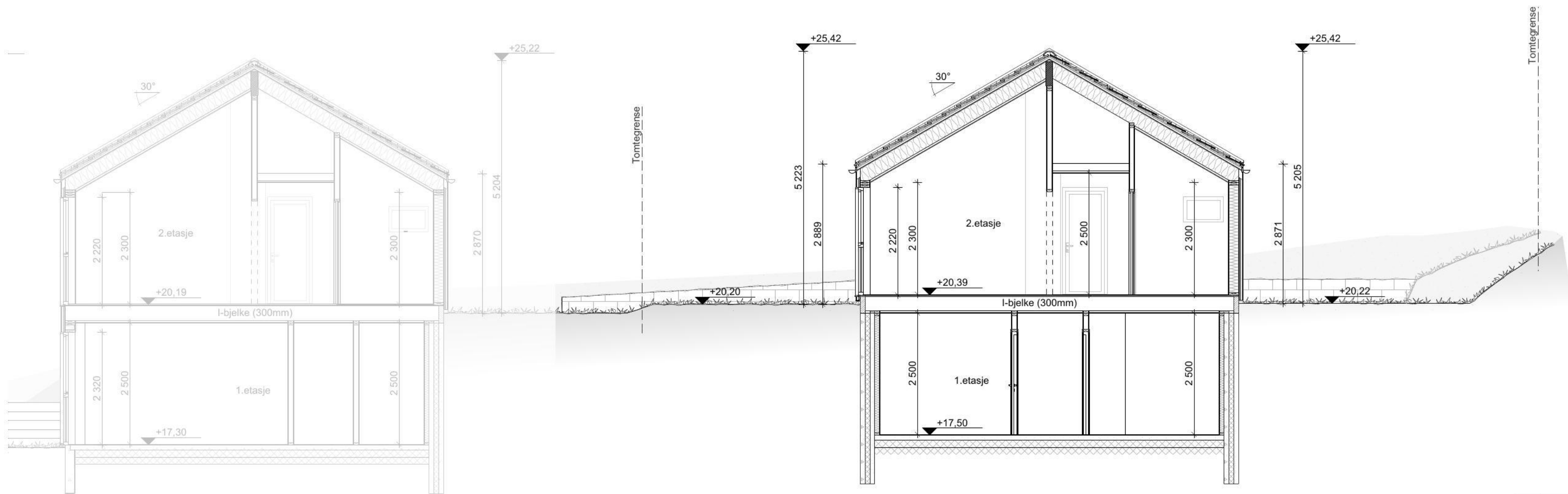
Snitt B-B bolig A
