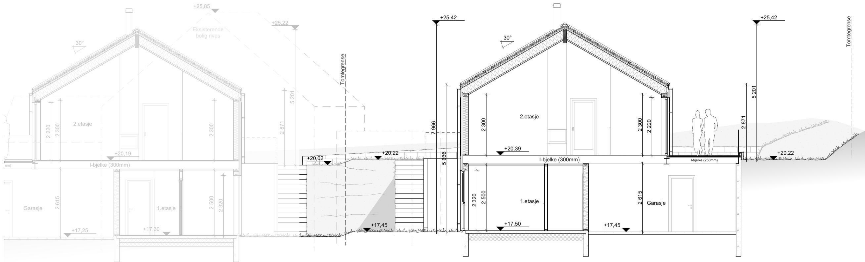
Snitt A-A bolig A
